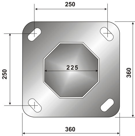
ПОДПЯТНИК 250
