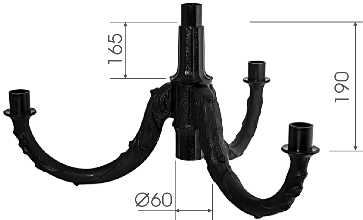
Система консолей "3+1" вверх
